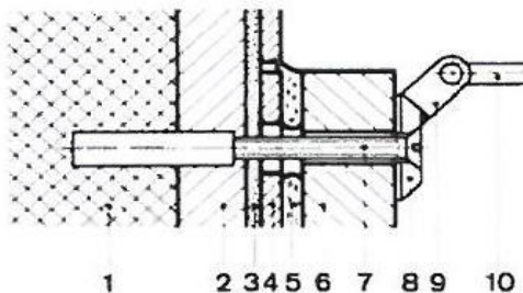
Détail de fixation avec grille rabattable
